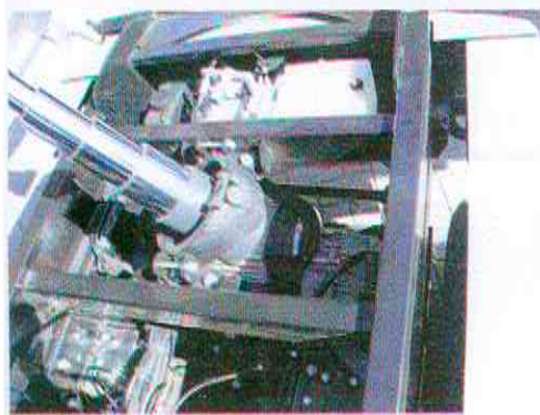
Bij de versie met tweewielaandrijving ligt de elektromotor met transmissie overdwars tussen de twee achterwielen.
